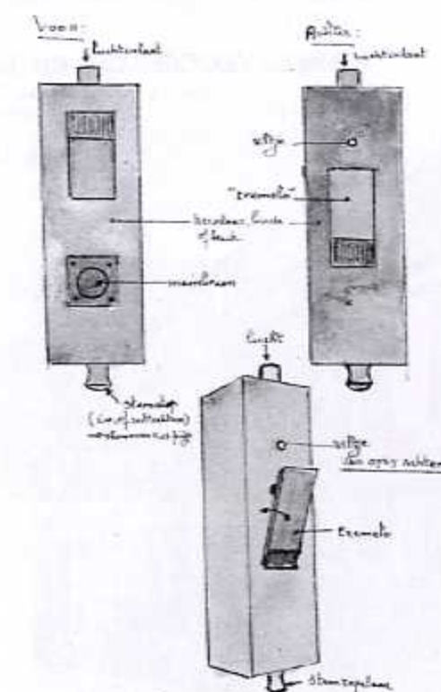
Schema orgelpijp dansorgel
